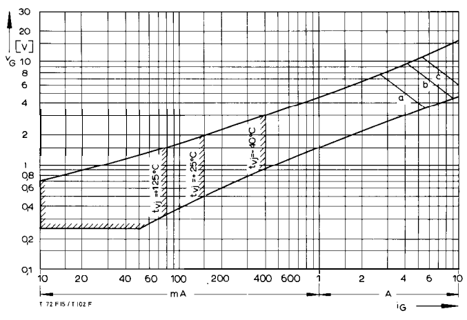
Bild/Fig. 19 Steuercharakteristik mit Zündbereichen/Gata Characteristic with triggering areas v_G = f(i_G) , V_o = 12 \text{ V}
